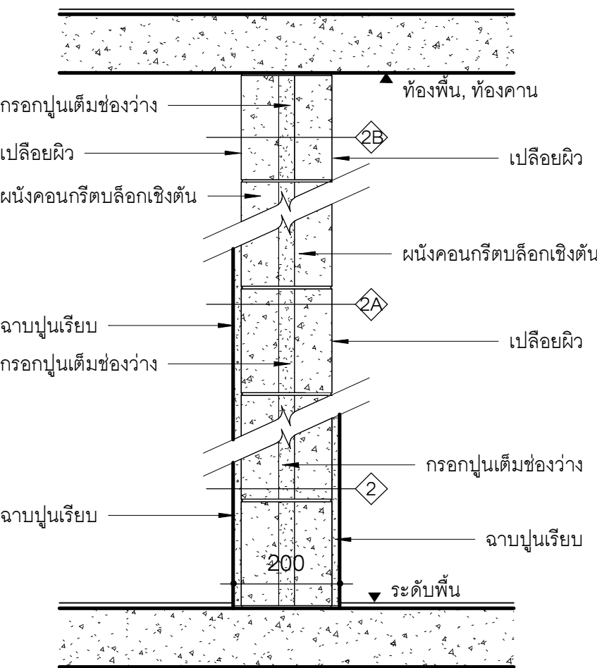
ผนังแบบที่ 2 ผนังคอนกรีตบล็อกเชิงตัน ทหนา 200 มม.
