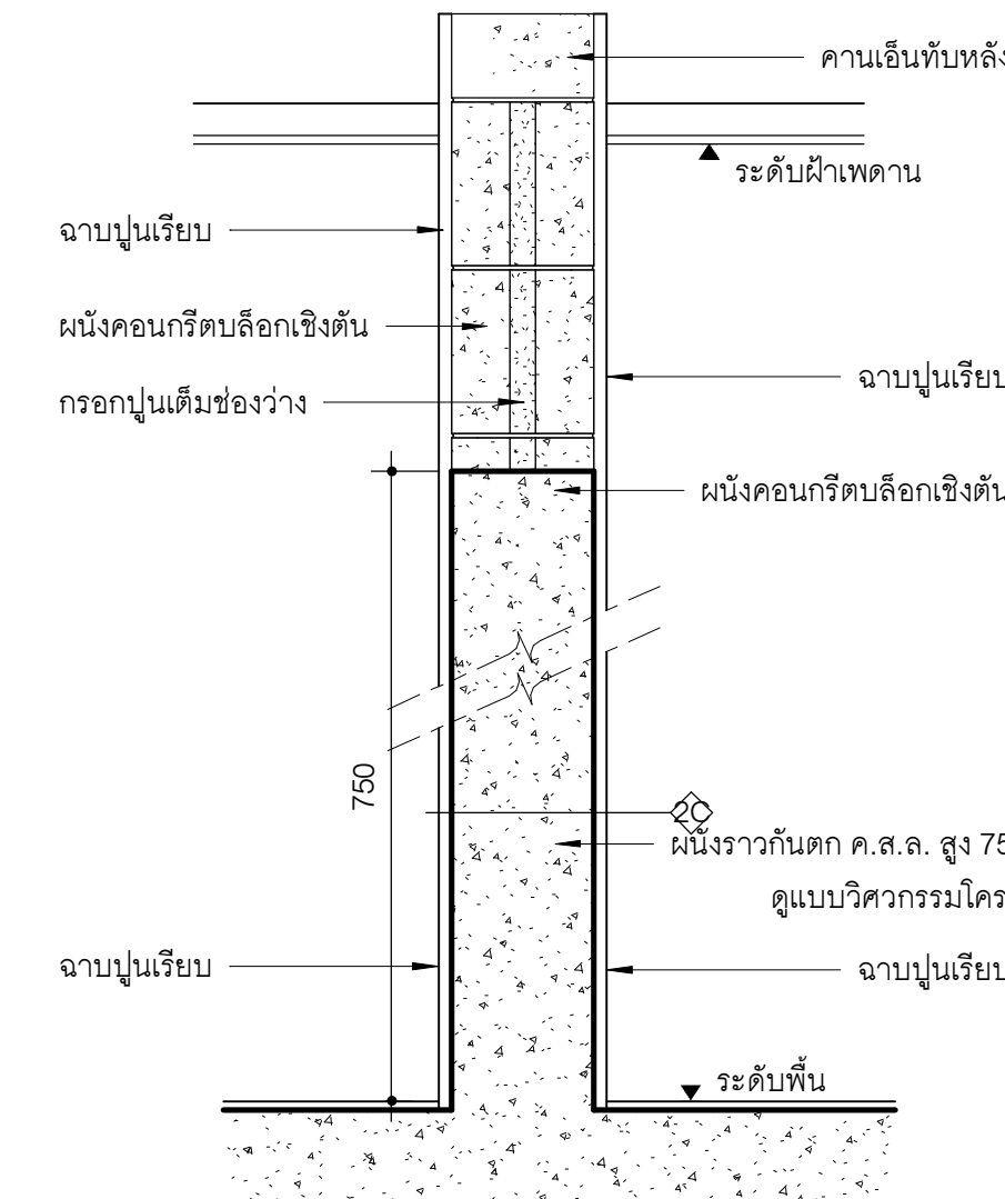
ผนังแบบที่ 5 ผนังคอนกรีตฉาบเรียบ ทหนา 200 มม.
