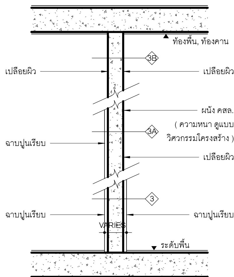
ผนังแบบที่ 3 ผนังคอนกรีตเสริมเหล็ก
